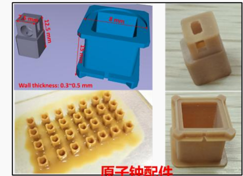
原子钟配件
